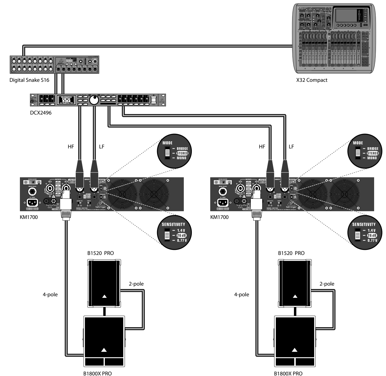
Vertical Bi-amping Bi-amplificación vertical Bi-amplification verticale Vertikales Bi-Amping Bi-amplificador Vertical
